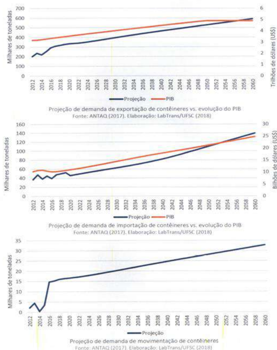
Figura 34 – Projeções de demanda de exportação, importação e de movimentação de contêineres
