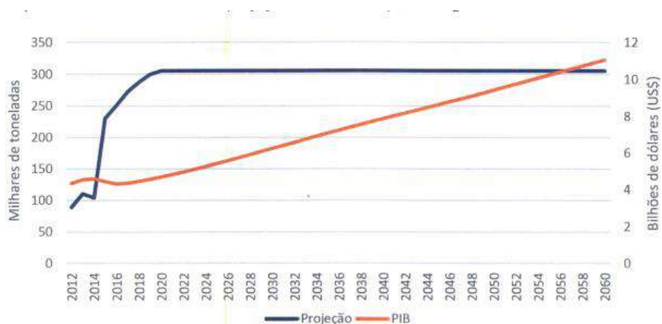
Figura 31 - Projeção de demanda de importação de trigo vs. evolução do PIB
